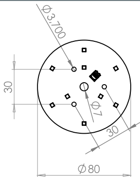
PCB-80-3030-9
